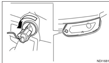
Přední směrové světlo
